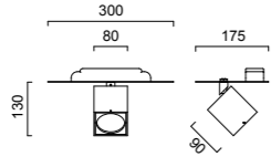
1 x HIT-TC-CE, 20 W, PGJ5 1,6 kg 15035.14 glanzweiß / glossy white / blanc brillant 15035.46 silbergrau / silver grey / gris-argenté
