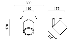
1 x HIT-TC-CE, 70 W, G8,5 2,2 kg 15046.14 glanzweiß / glossy white / blanc brillant 15046.46 silbergrau / silver grey / gris-argenté
