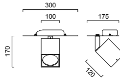
1 x HIT-TC-CE, 70 W, G8,5 2,2 kg 15037.14 glanzweiß / glossy white / blanc brillant 15037.46 silbergrau / silver grey / gris-argenté
