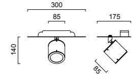
1 x HIT-TC-CE, 20 W, PGJ5 1,6 kg 15061.14 glanzweiß / glossy white / blanc brillant 15061.46 silbergrau / silver grey / gris-argenté
