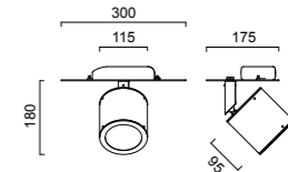
1 x HIT-TC-CE, 70 W, G8,5 2,2 kg 15063.14 glanzweiß / glossy white / blanc brillant 15063.46 silbergrau / silver grey / gris-argenté
