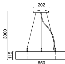
Pendelleuchtenarmatur mit Baldachin, chrom (ohne Leuchtschirm) Pendant light fixture with canopy, chrome (without shade)
